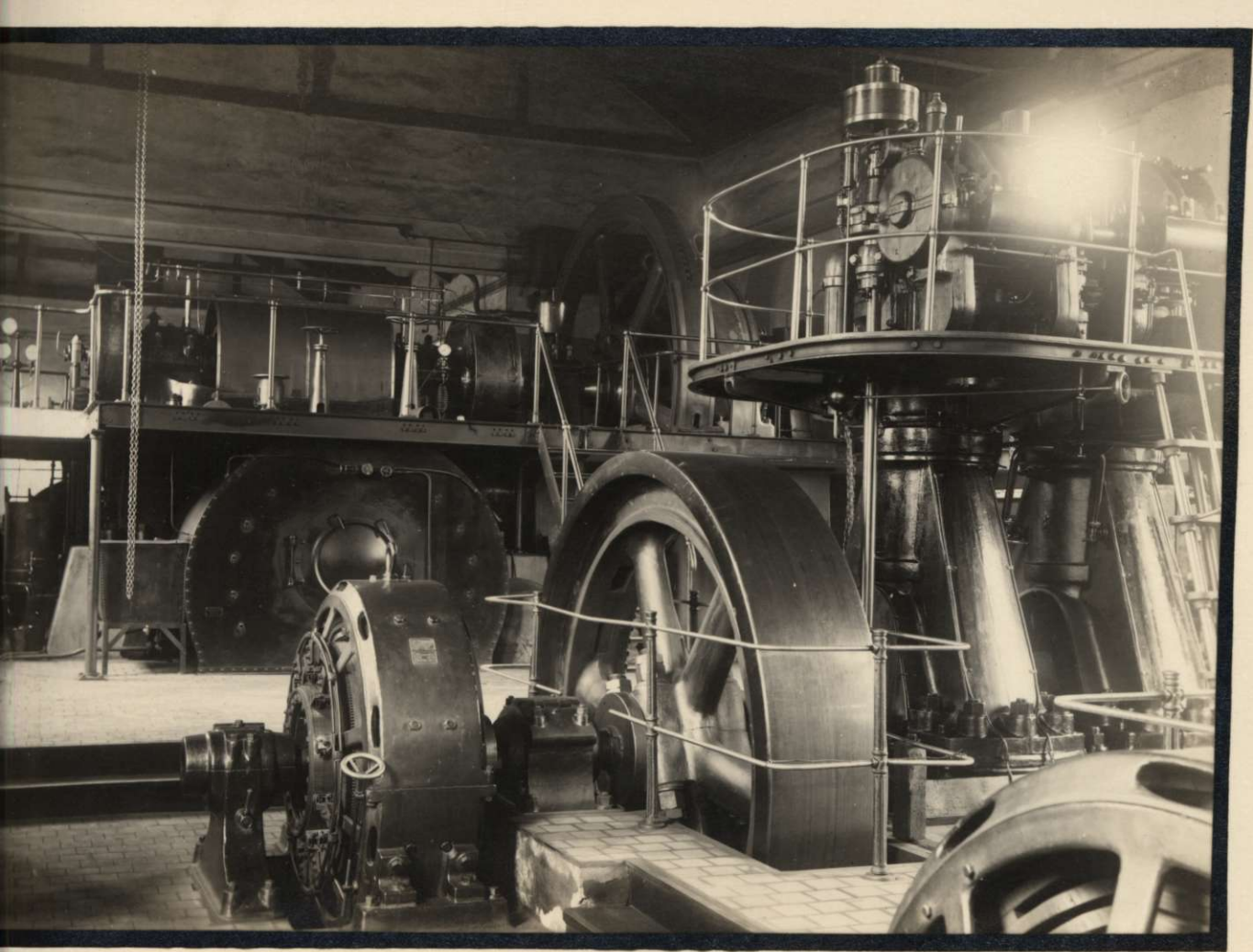
A villamosmű 560 L. E. gőzegysége.
