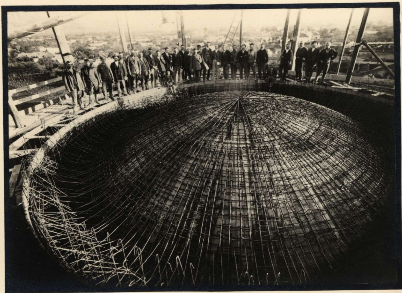
A torony vízmedence-fenék vasszerelése.
