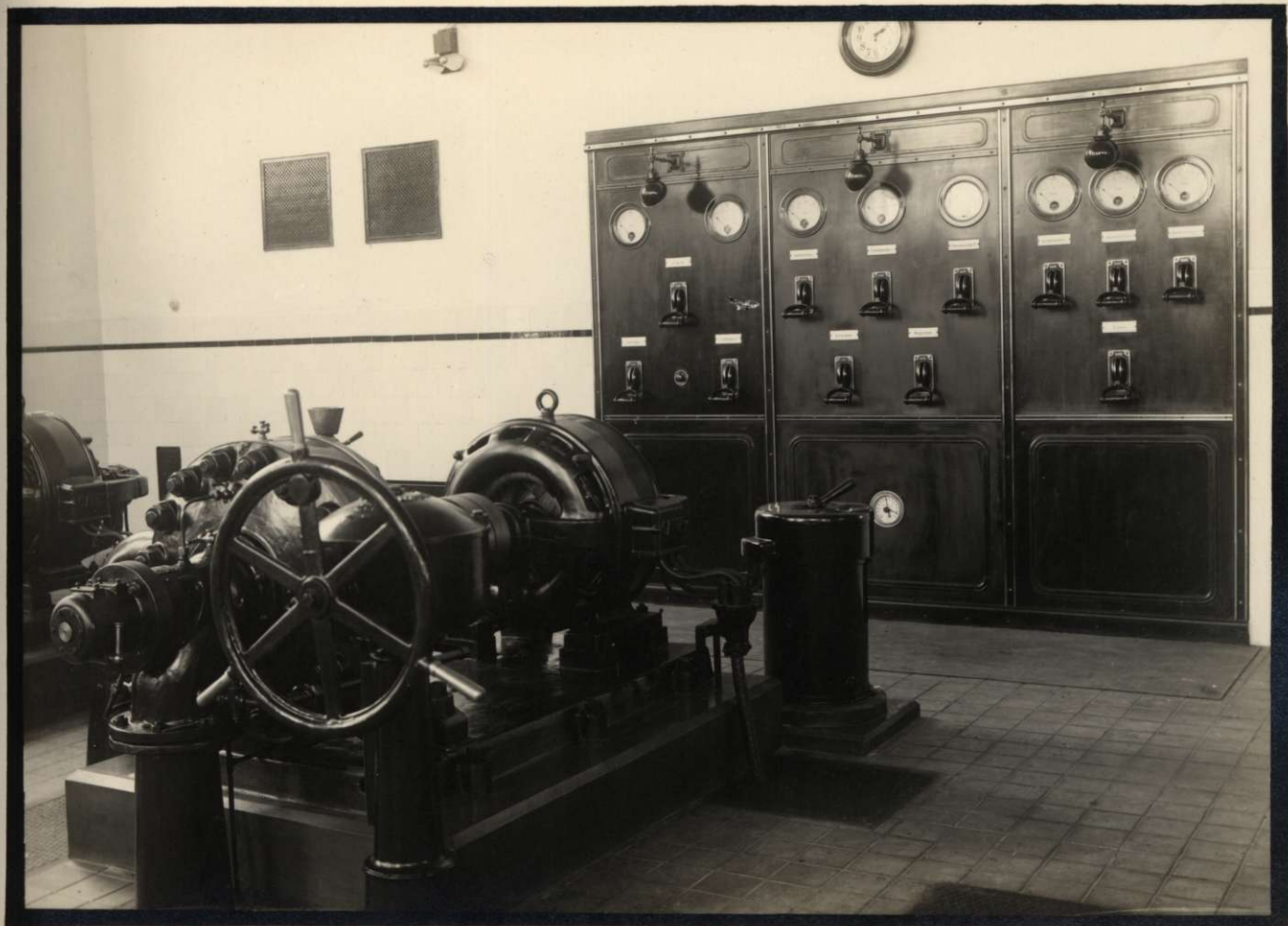
Tisztavíz-szivattyúk és kapcsoló-tábla. Szállították: Ganz és Társa és Ganz-féle Vill. r.-t.
