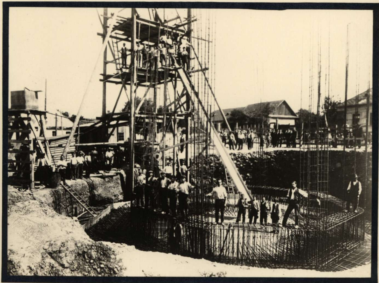
Víztorony vasbeton-alap szerelése.
